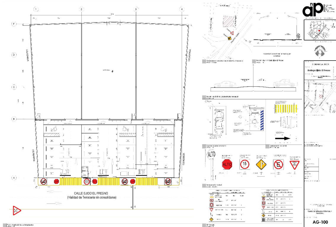
IMAGEN 92.- Plano Revisión de accesos autorizado. Fuente. Departamento de Ingeniería Vial
