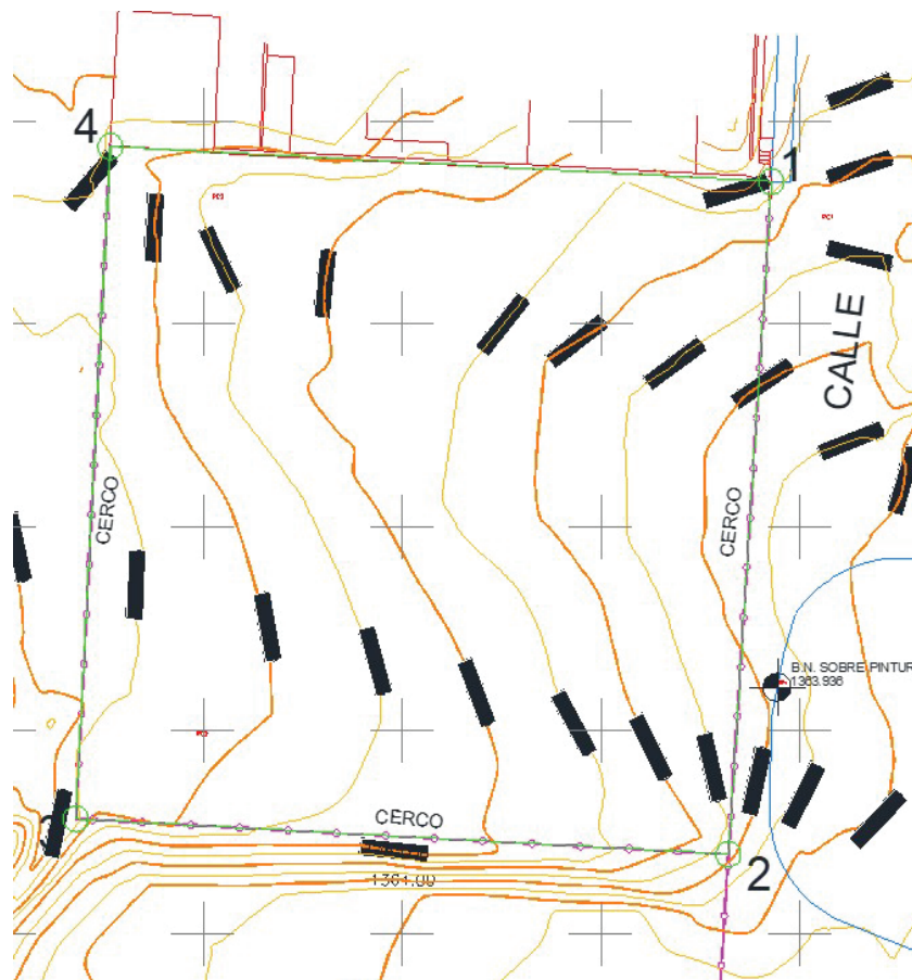
IMAGEN 27.- Levantamiento Topográfico. Fuente: Ing. Rivera Abud.
