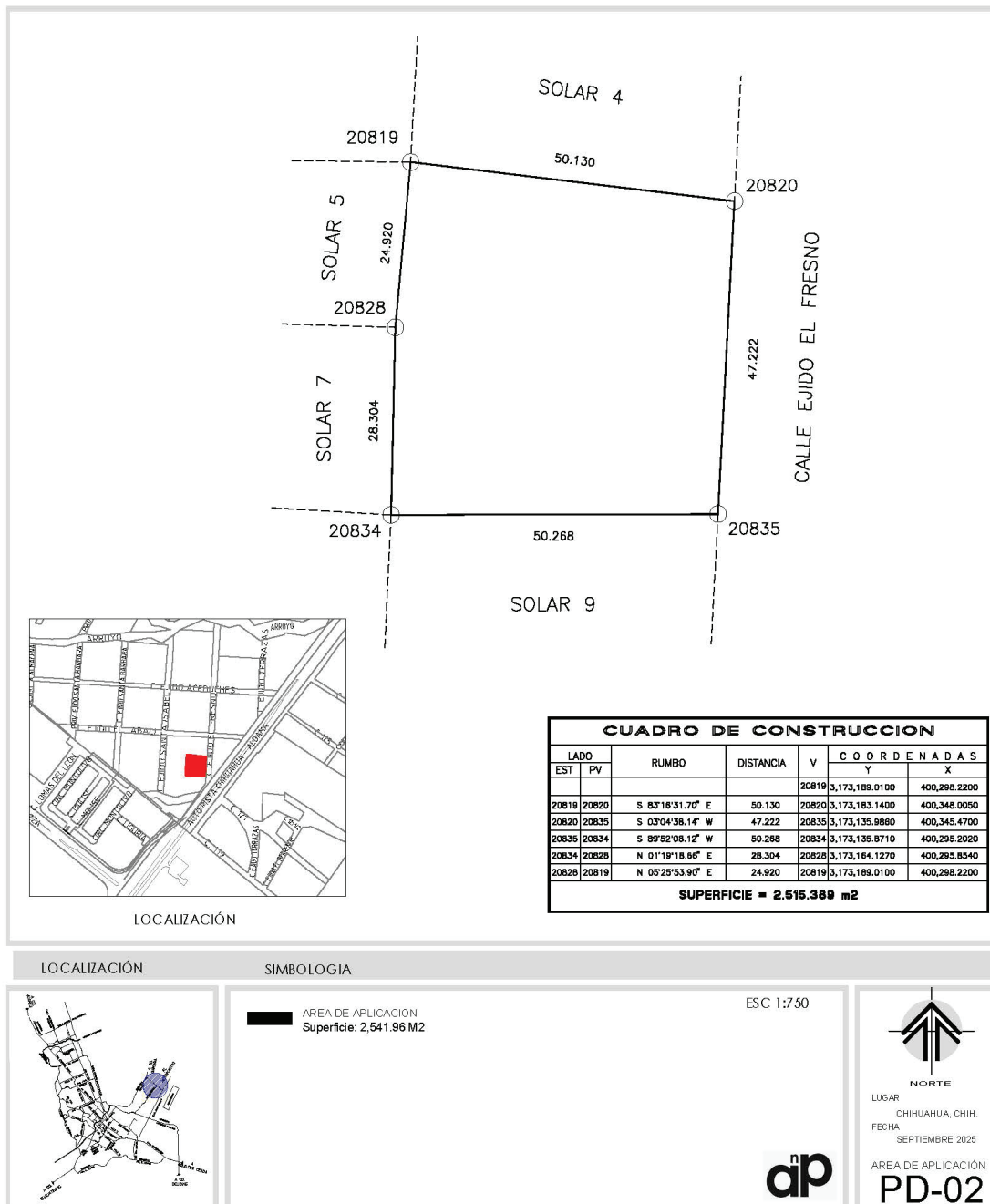
IMAGEN 4.- Cuadro de construcción área de aplicación. Fuente: Elaboración propia.
