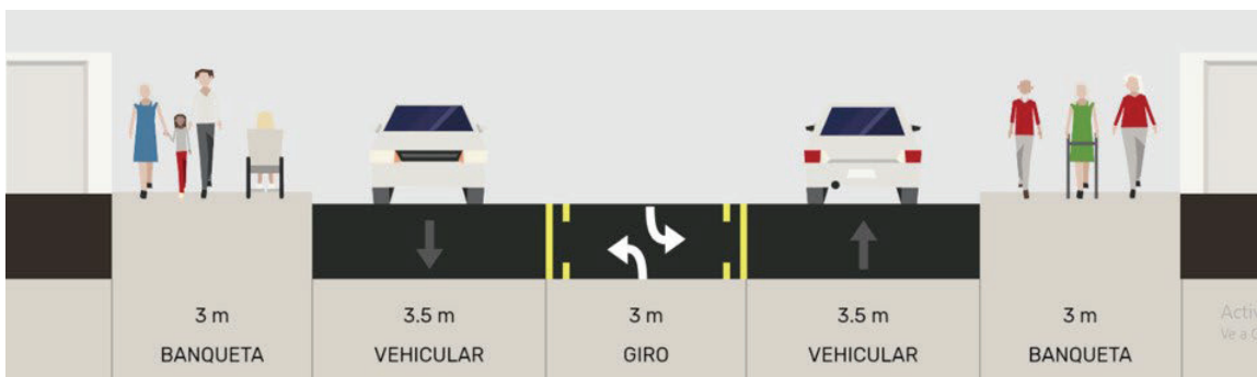
IMAGEN 55.- Sección vial Calle Libia. Fuente: PDU del Centro de Población Chihuahua Visión 2040 7ª actualización.
