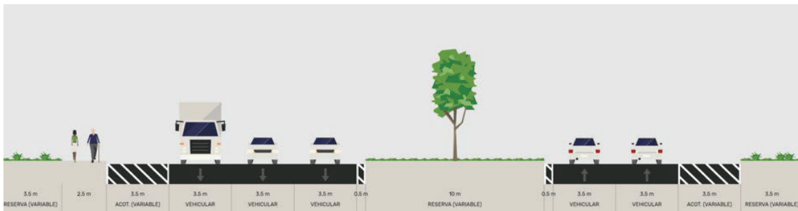
IMAGEN 89.- Sección Carretera Chihuahua-Aldama. Fuente: PDU del Centro de Población Chihuahua Visión 2040 7ª actualización.
