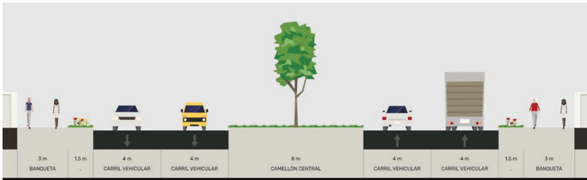
IMAGEN 56.- Sección vial Blvd. Romanzza. Fuente: PDU del Centro de Población Chihuahua Visión 2040 7ª actualización.
