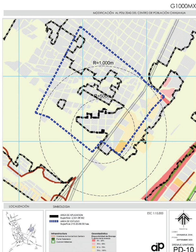
IMAGEN 61.- Infraestructura de drenaje sanitario en el área de estudio. Fuente: PDU de la ciudad de Chihuahua: Visión 2040.
