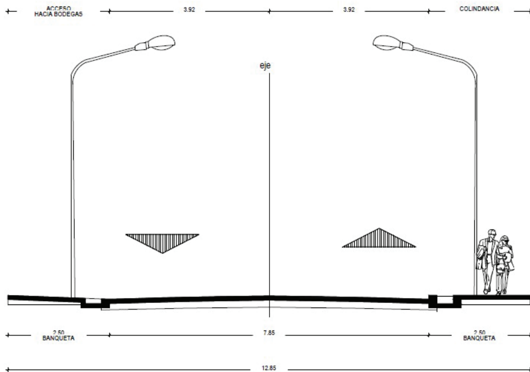
IMAGEN 57.- Sección calle Ejido El Fresno. Fuente. Elaboración propia.
